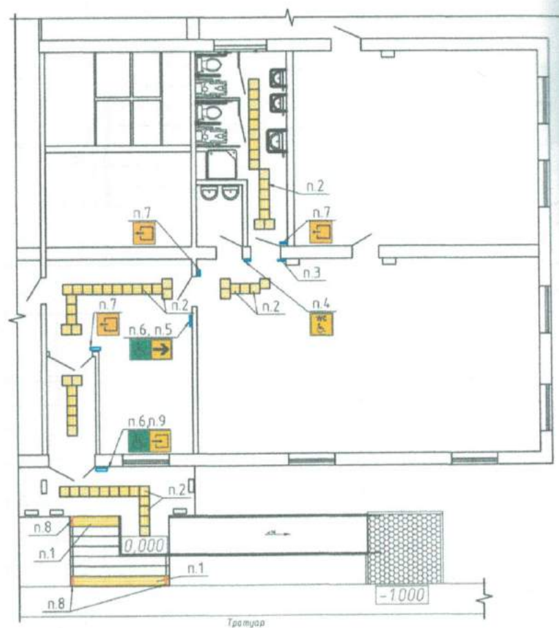
Схема расположения тактильных указателей
